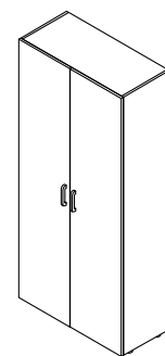
ART.101 90x42x198h
