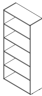
ART.100 90x40x198h
