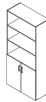
ART.103 90x42x198h
